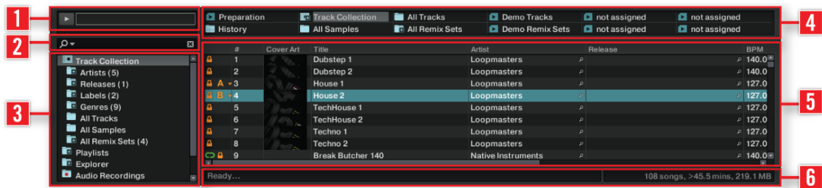
TRAKTOR's Browser
