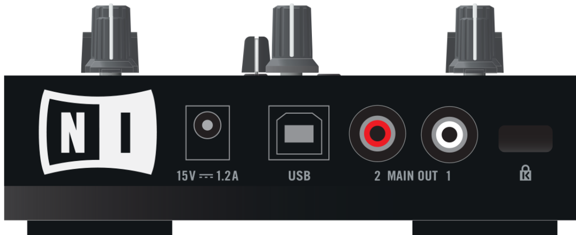
Le panneau arrière du Z1
